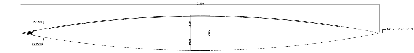
V1 (FBX AR4 ENV CLD ROF R278 SUB) SECTION-V1 1/100
